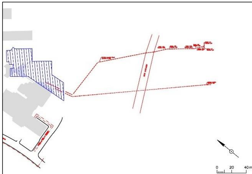
FIGURE 18 : PLAN DES INFRASTRUCTURES CIVILES DANS LE SECTEUR CIBLÉ PAR LES TRAVAUX DE CONSTRUCTION DE L'ESPACE RIOPELLE, (DONNÉES : MUSÉE NATIONAL DES BEAUX-ARTS DU QUÉBEC).
